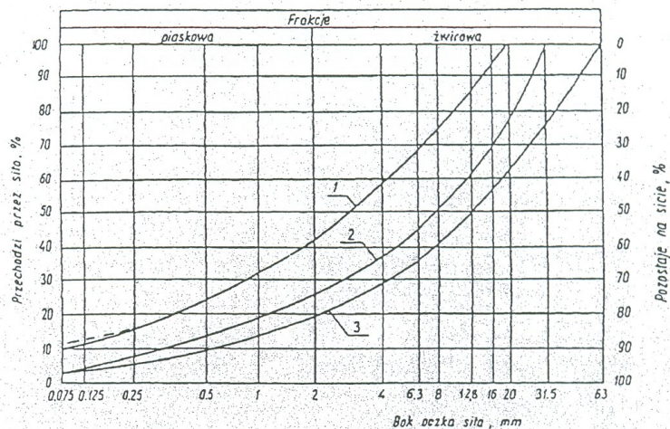
Rysunek 1. Pole dobrego uziarnienia kruszyw przeznaczonych na podbudowę wykonywane metodą stabilizacji mechanicznej 1-2 kruszywo na podbudowę zasadniczą.
