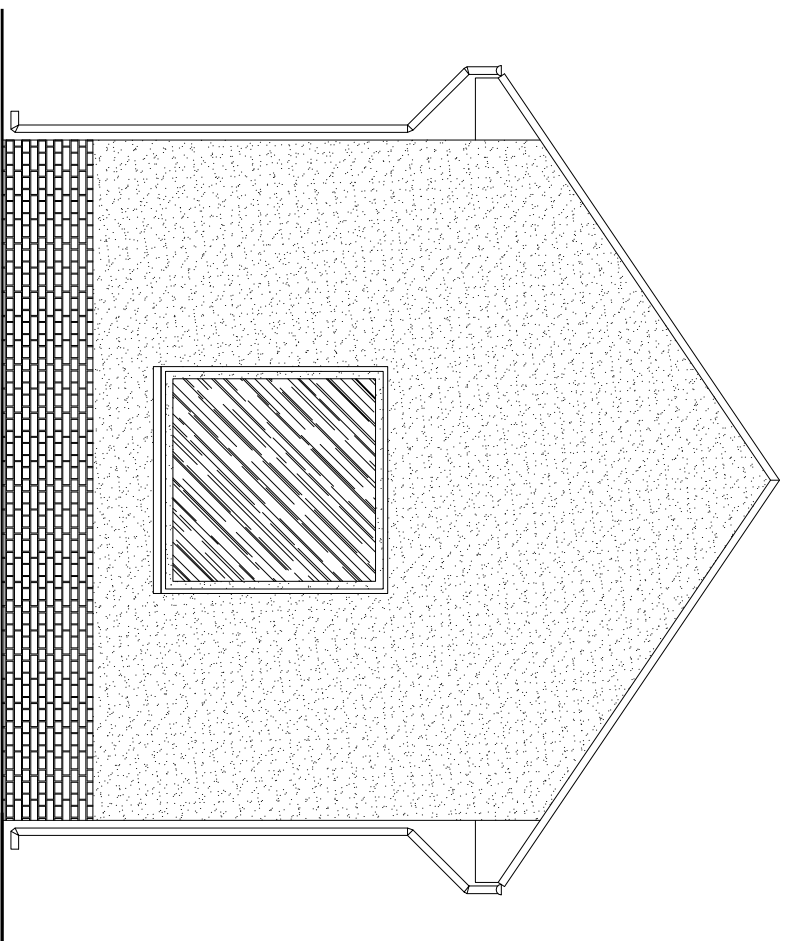
ELEWACJA ZACHODNIA
