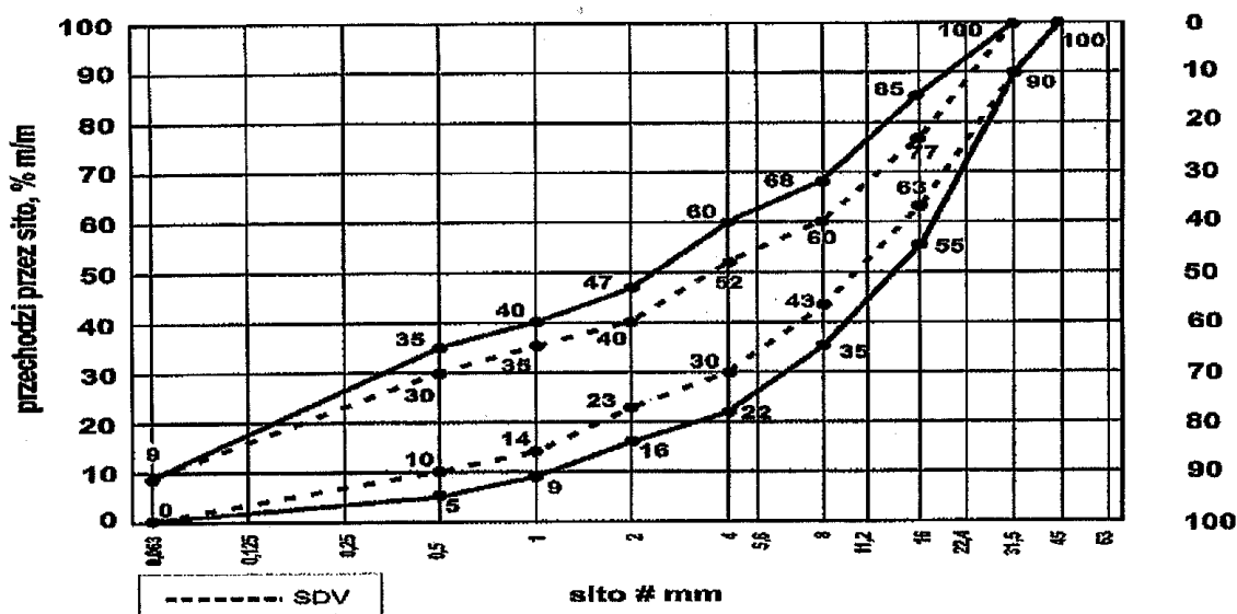
Rysunek 2. Uziarnienie mieszanki niezwiązanej 0/31,5 do nawierzchni
