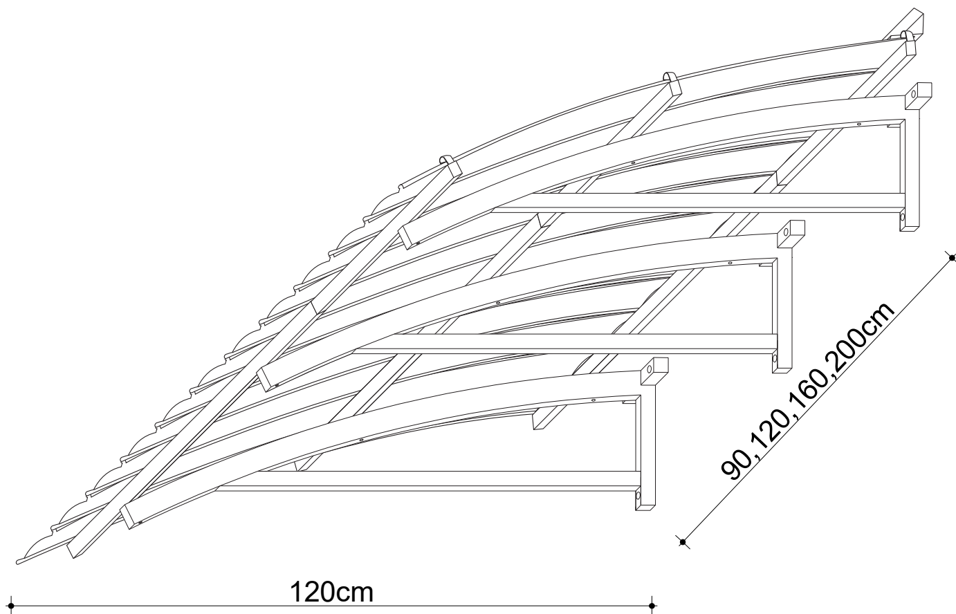
ZADASZENIE NAD WEJŚCIEM DO BUDYNKU SZEROKOŚCI WG. RYSUNKU ELEWACJI
