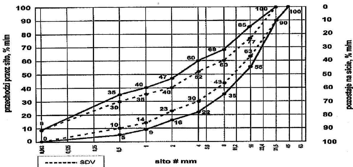
Rysunek 2. Uziarnienie mieszanki niezwiązanej 0/31,5 do nawierzchni
